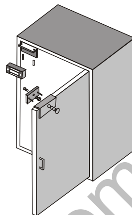
Установка с UL уголком
